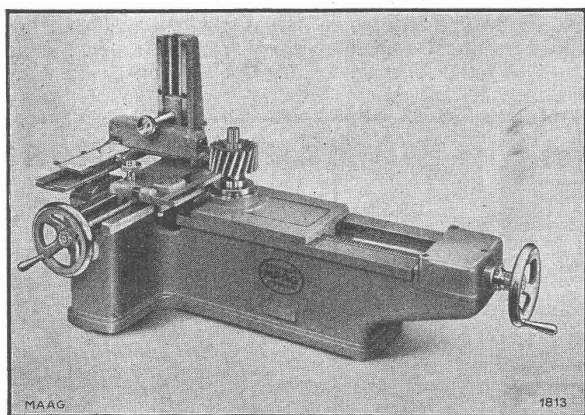
MAAG-Flankenprüfgerät, Typ FPV-40, zur Kontrolle des Zahnprofils an Stirn- und Schraubenzähnen.
