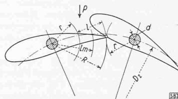
Abb. 17. Schematische Skizze zur Berechnung des Drehmomentes einer Leitschaufel in geschlossener Stellung
