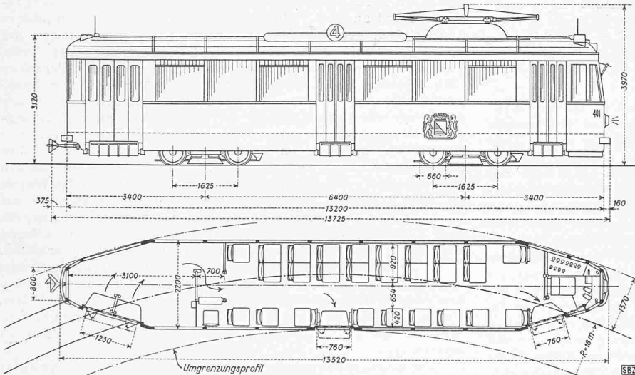
Abb. 6. Vierachsiger Strassenbahnwagen Reihe 401 der St. St. Z. — Typenskizze 1:120 Leichtbauweise, Tara 12,9 t, 27 Sitz-, 73 Stehplätze. Platzgewicht 129 kg
