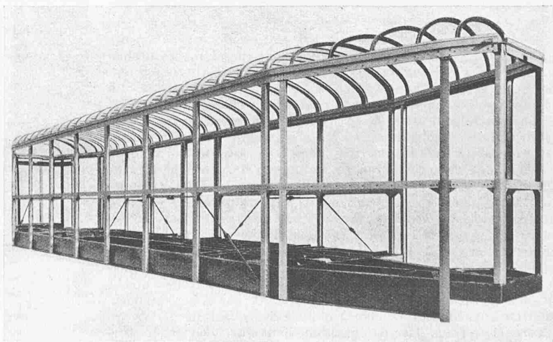
Abb. 7. Das 13,2 m lange Kastengerippe, Schweiz. Wagons- und Aufzügefabrik Schlieren
