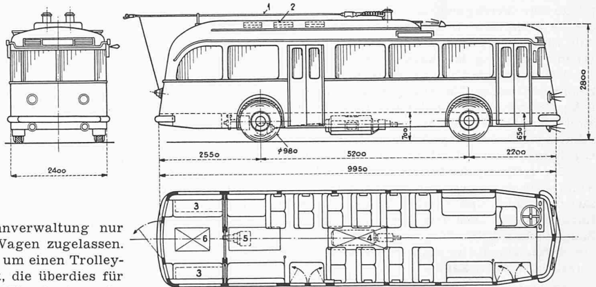
Abb. 4. Typenskizze des Trolleybus. — 1 Trolley, 2 Widerstände, 3 Hochspannungs-Apparatur, 4 Motor, 5 Kompressor, 6 Akkumulatoren
