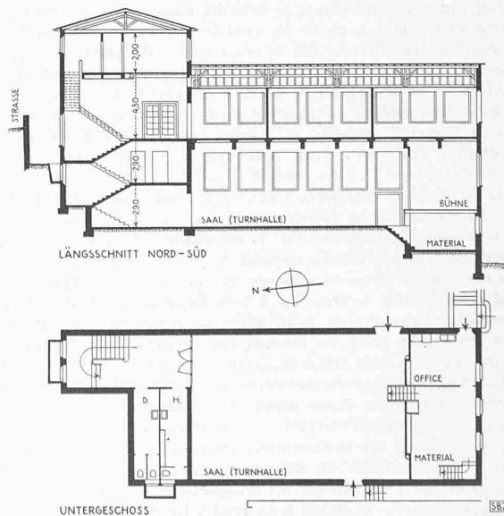
Abb. 17 u. 18. Längsschnitt und Untergeschoss-Grundriss 1: 400
