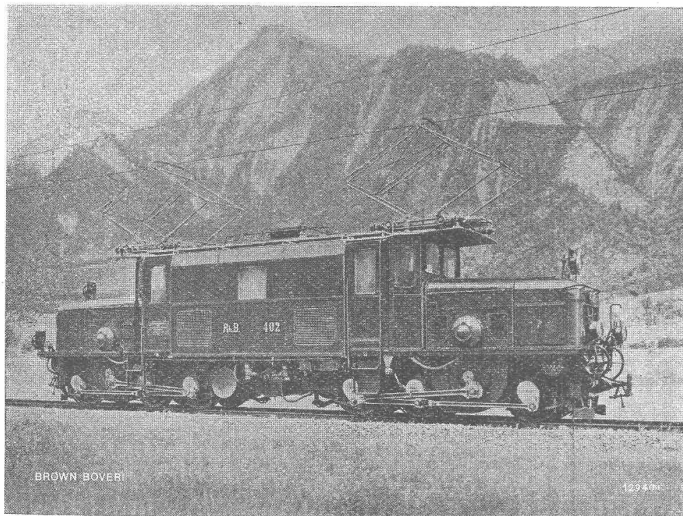
Einphasenstrom-Lokomotive, Typ C-C für die Rhätische Bahn 2 × 600 PS, 10000 Volt Fahrdrachtspannung, Frequenz 16 \frac{2}{3} Geschwindigkeit 30 bis 45 km/h, Spurweite 1 m.
