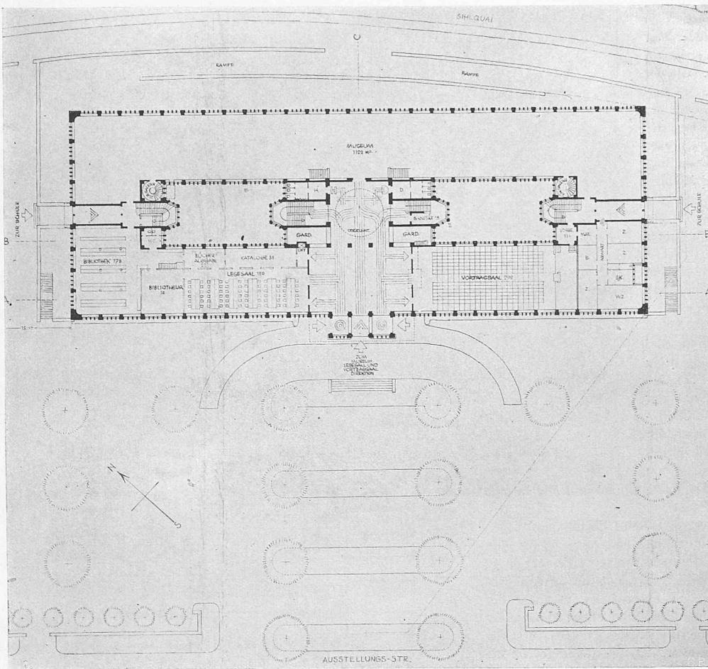
Fassade gegen die Ausstellungsstrasse, Schnitt und Erdgeschoss-Grundriss. — Masstab 1 : 800.
