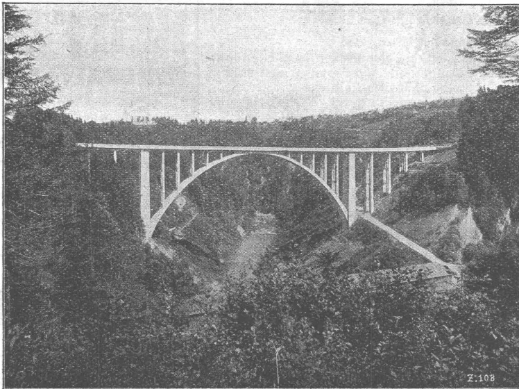
Hundwillertobelbrücke im Kanton Appenzel A. Rh. Spannweite des Bogens 105 m.
