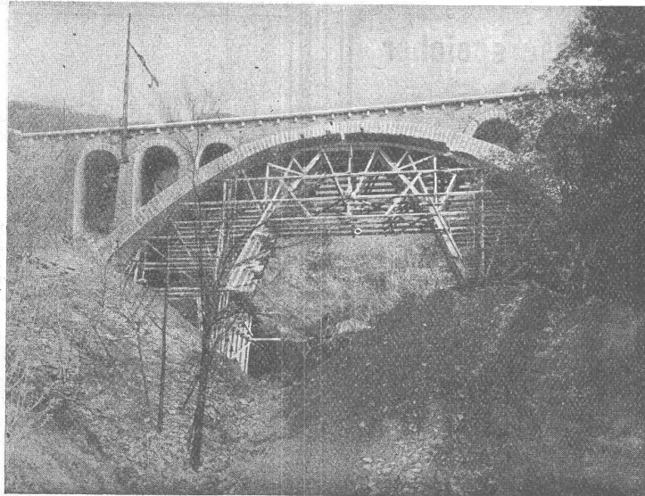
S. B. B., Monte Ceneri-Linie, Selvaccia-Brücke, zweigeleisig, 42,20 m l. W.
