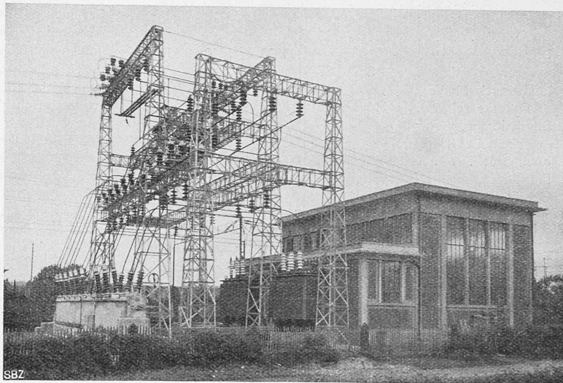
Freiluft-Unterwerk Coaraze-Nay der Midi-Bahn bei Pau (Text siehe Seite 13).
