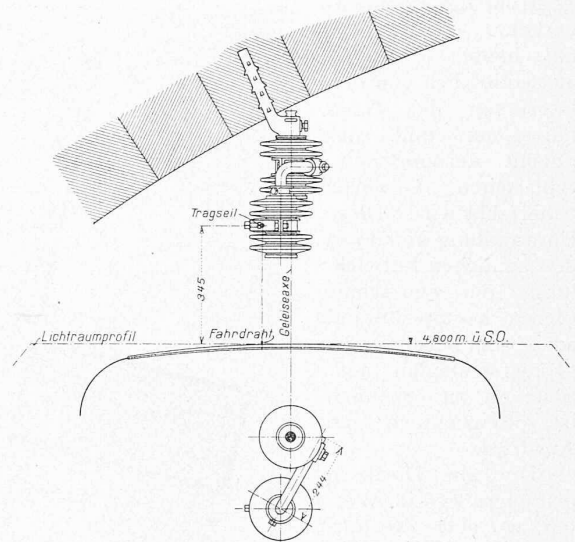
Abb. 41. Tunnel-Zwischenstützpunkt. — Masstab 1 : 20.
