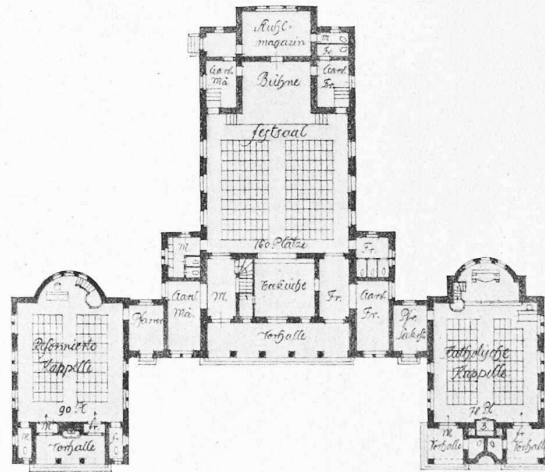
Saalbau, Grundriss und Nordwestfassade 1:600.
