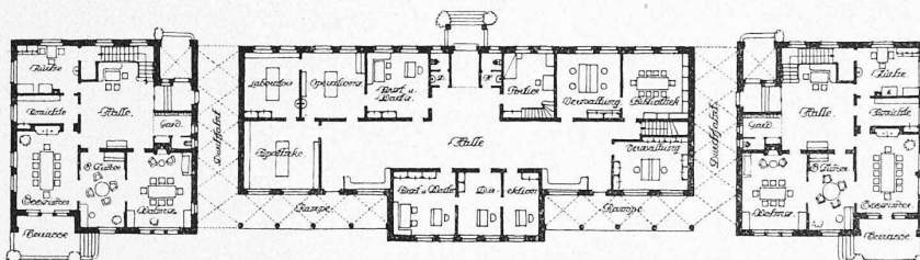
Entwurf Nr. 25. — Architekten Gebr. Messmer , Zürich. — Verwaltungsgebäude.
