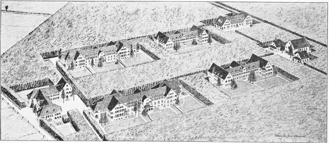
II. Rang. Entwurf Nr. 8. Motto „Sü, Fräischamaing“. Architekt Richard von Murali, Zürich. Vogelschau und Lageplan: 1:2000.
