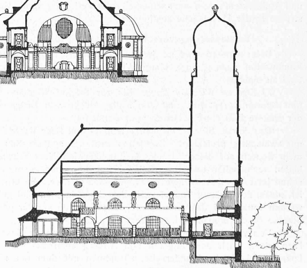
Quer- und Längsschnitt. — Masstab 1:600.
