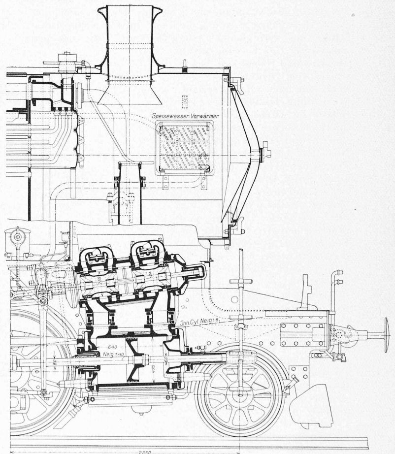
Abb. 5 und 6. Querschnitte und Längsschnitte der Doppel-Zwilling-Lokomotive C \frac{5}{6} . — Masstab 1 : 35.
