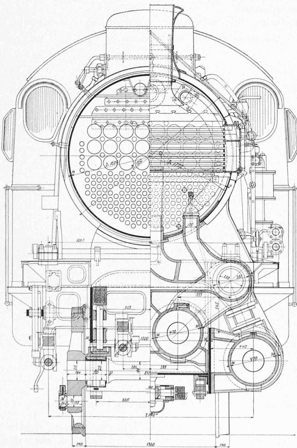
Abb. 5 und 6. Querschnitte und Längsschnitte der Doppel-Zwilling-Lokomotive C \frac{5}{6} . — Masstab 1 : 35.
