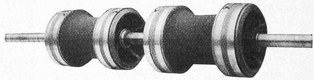
Abb. 9. Doppelkolbenschieber.
