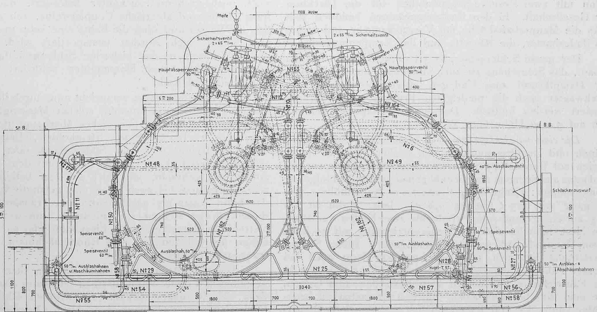
Querschnitte des Schleppdampfers « France »: Abb. 7 Spant 56; Abb. 8 Spant 73 und Abb. 9 Spant 91 (von vorn gesehen). Masstab 1 : 60.
