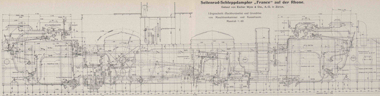
Ganze Länge des Maschinenraumes 18,500 Starb. Länge des Maschinen- und der Kesselraumes 28,500
