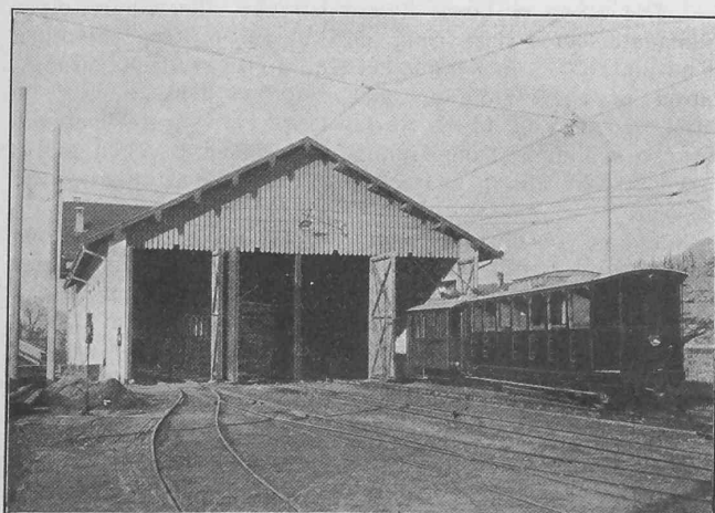
Abb. 6. Aigle-Leysin-Bahn. — Fahrdepot.
