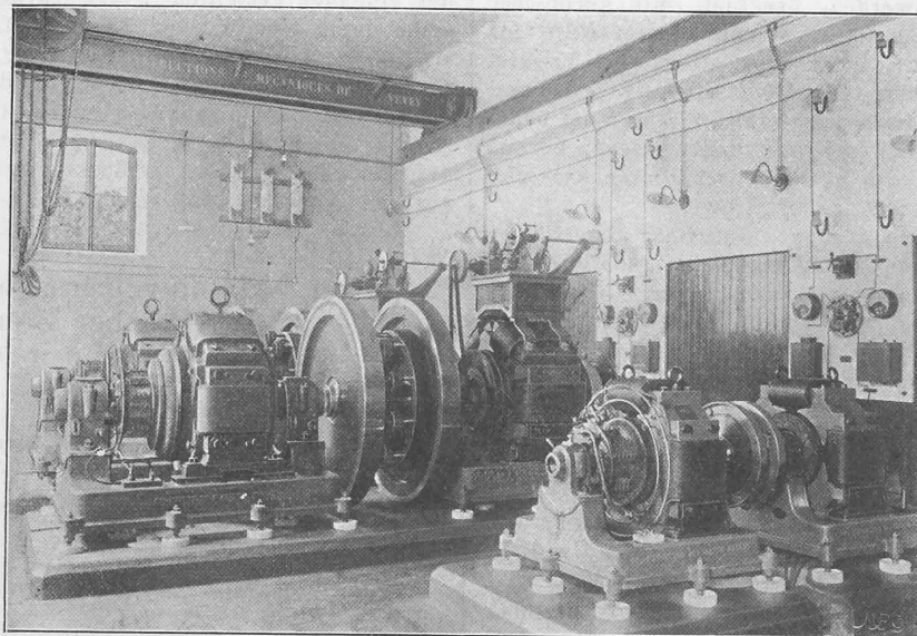
Abb. 8. Aigle-Leysin-Bahn. — Innenansicht der Umformerstation.
