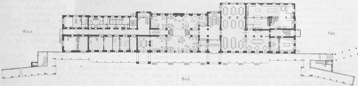
Abb. 5. Grundriss vom Erdgeschoss. — Masstab 1:750.
