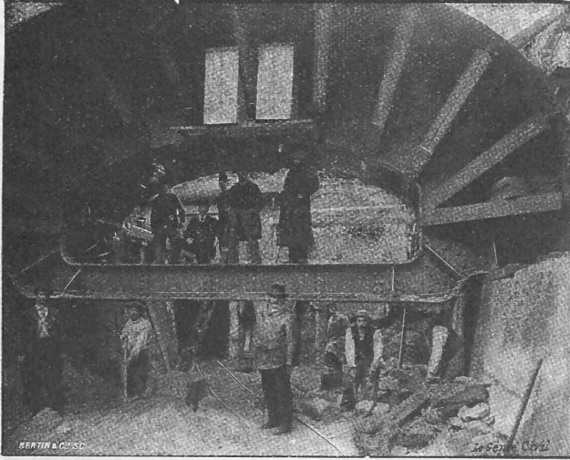
Abb. 5. Ansicht des Chagnaud'schen Schildes.
