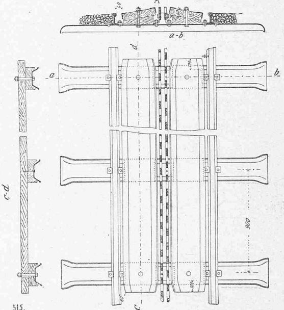
Generosobahn. — Oberbau. Fig. 35—37. Wegübergang
