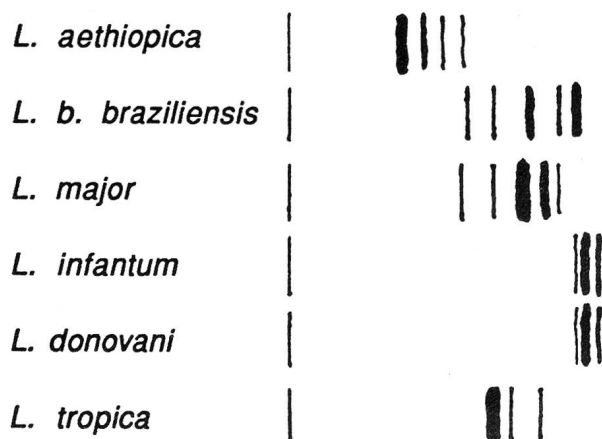
Abb. 1: Schematische Darstellung des Isoenzymmusters der Glucosephosphat-Isomerase (GPI) bei verschiedenen Leishmania -Arten: L. aethiopica (L 100), L. braziliensis (LEM 781), L. major (LEM 769), L. infantum (LEM 75), L. donovani (DD 8), L. tropica (K 27)
