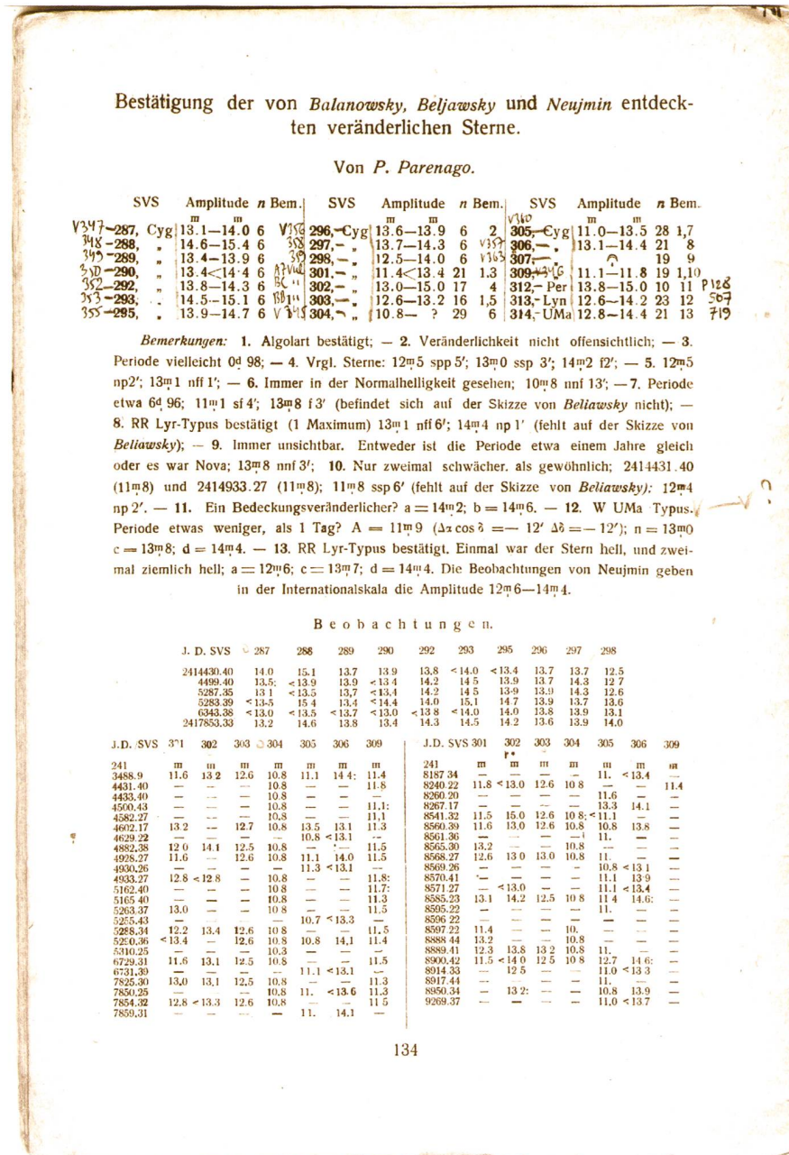
Abb. 2: Der Anfang des Beitrages von Paul Parenago in PZ 4.134, in dem er unter anderem auch die Veränderlichkeit der von Beljawsky entdeckten Sterne bestätigt. Hinter der Bezeichnung SVS 303 verbirgt sich der uns interessierende BB Vul.
