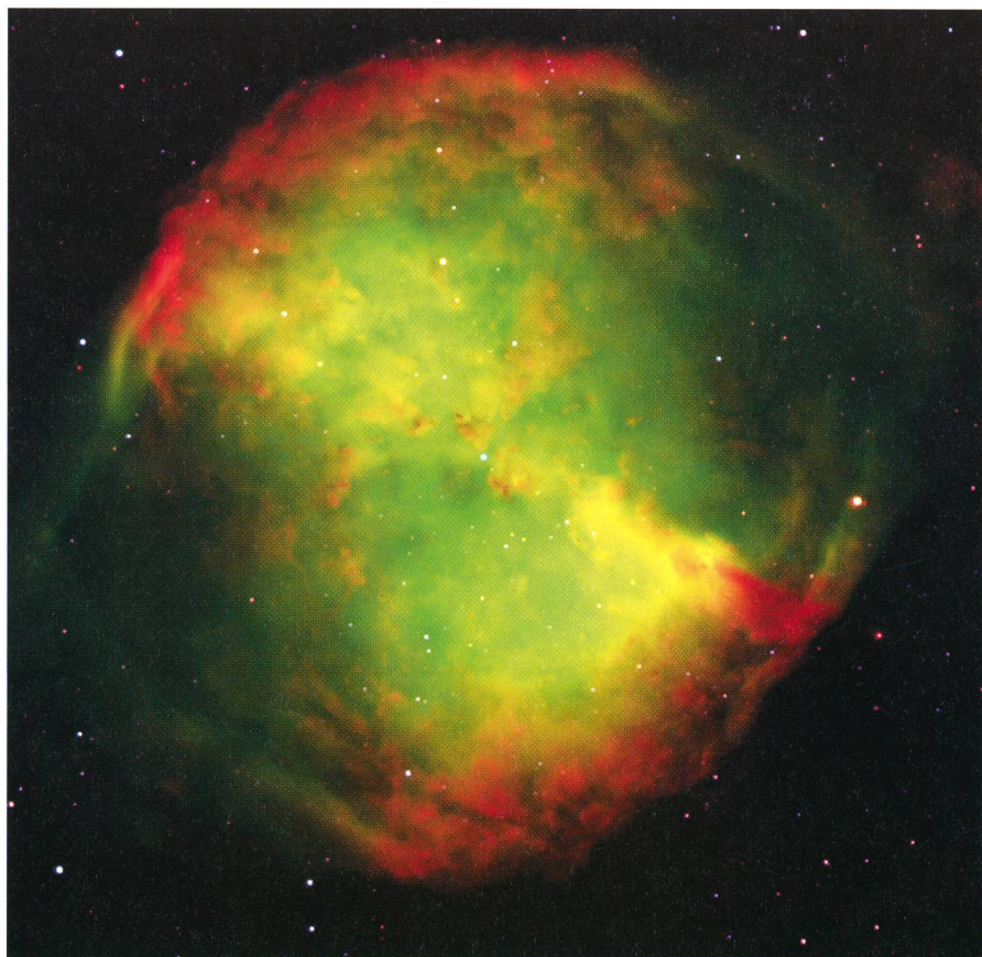
Fig. 13: La nébuleuse planétaire NGC 6853 (M27)(Photo VLT).
