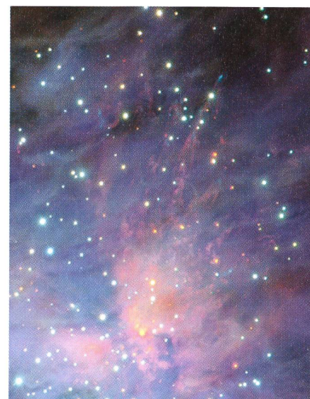
Fig. 1bis: Détail de la nébuleuse d'Orion. C'est la plus proche (à environ 1500 AL) et la mieux étudiée des régions de formation de nouvelles étoiles. (Image VLT)
