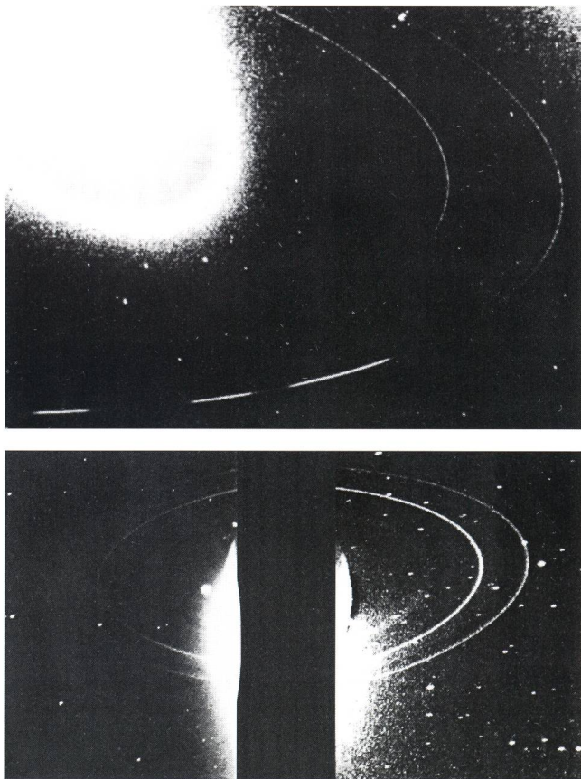
Figures 2a,b) Les anneaux de Neptune vus par Voyager 2. Le soleil se trouve dans le dos de la caméra; et Neptune est surexposée pour pouvoir faire apparaître les anneaux. (Source [1]).
