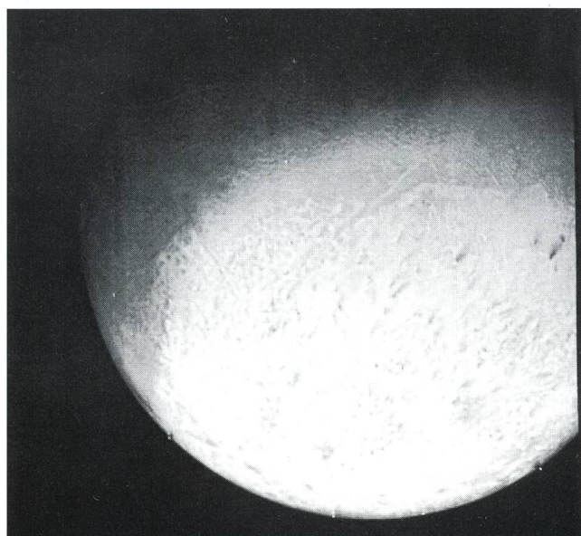
Figure 3) Le satellite Triton. Image, prise le 24.8.1989 d'une distance de 530000 km avec une résolution de 10 km, constituée à partir d'images captées à travers les filtres vert, violet et ultraviolet. (Source [1]).
