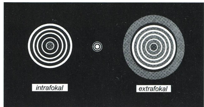
Abb.5: Mit Hilfe des Computers schematisch gezeichnet die intra- und extrafokalen Beugungsbilder von 75 und 105 SDHF bei 100- bzw. 140-facher Vergrößerung.
