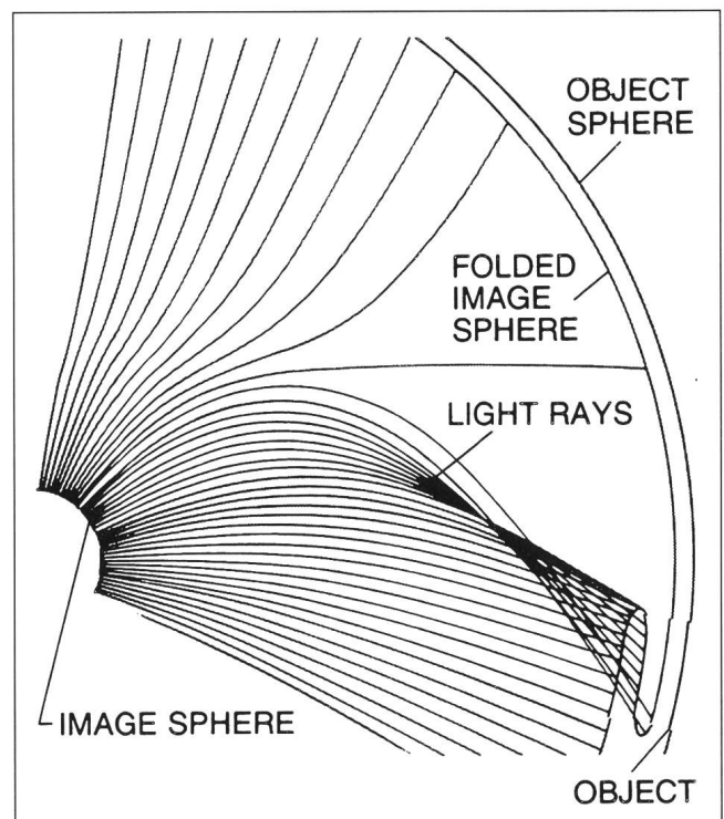
Figur 5. Ausbreitung von Lichtstrahlen zwischen Objekt- und Bildsphäre in einem Medium, welches starke Schwankungen des Brechungsindex aufweist. Da angrenzende Lichtstrahlen stetig ineinander übergehen müssen, tauchen mehrfache Bilder immer in ungerader Anzahl auf. Verfolgt man die Strahlen, von unten anfangend, so sieht man, wie das untere Bild aufrecht erscheint, das mittlere steht auf dem Kopf und das obere ist wieder aufrecht, obgleich dieses Bild in der Vertikalen oft stark komprimiert wird. [nach TAPE (3)]
