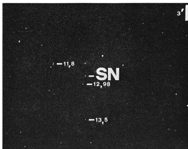
Aufnahme von F. SEILER vom 13. Juni im Newton-Primärfokus f = 1800 mm, \varnothing = 300 mm, 5 Minuten auf Ilford HPS.
