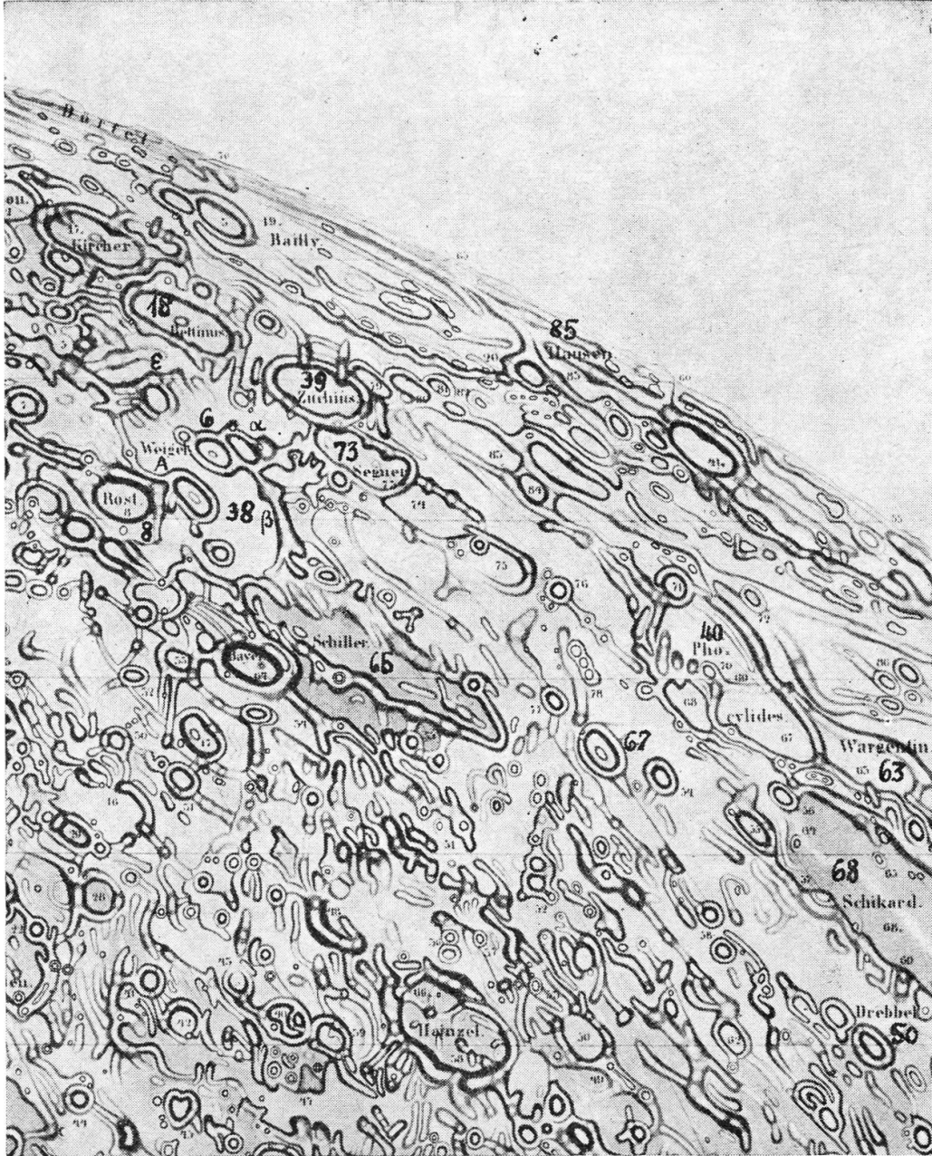
Abb. 2 Ausschnitt aus dem Mondatlas von Lohrmann mit der vom Verfasser als «Regio solitudinis» bezeichneten Mondlandschaft. Die besprochenen Formationen sind so weit als möglich nummeriert.
