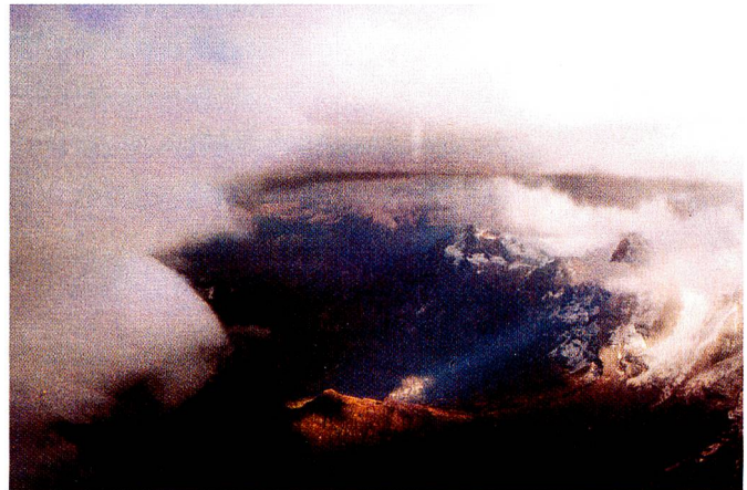
Abb. 12 Im kräftigen Abwindbereich des Rotors.
