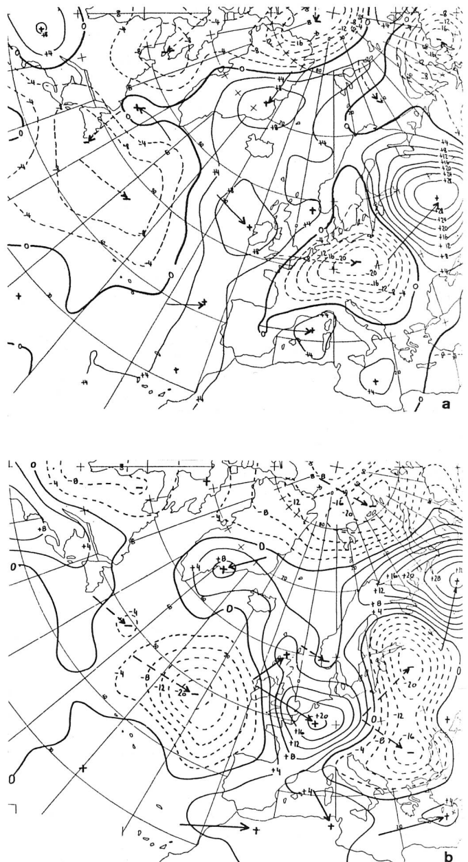
Abb. 8 24stündige Änderungen der relativen Topographie 500/1000 hPa in gpdam über Europa. a) 13. 12., 1 Uhr MEZ b) 14. 12., 1 Uhr MEZ
