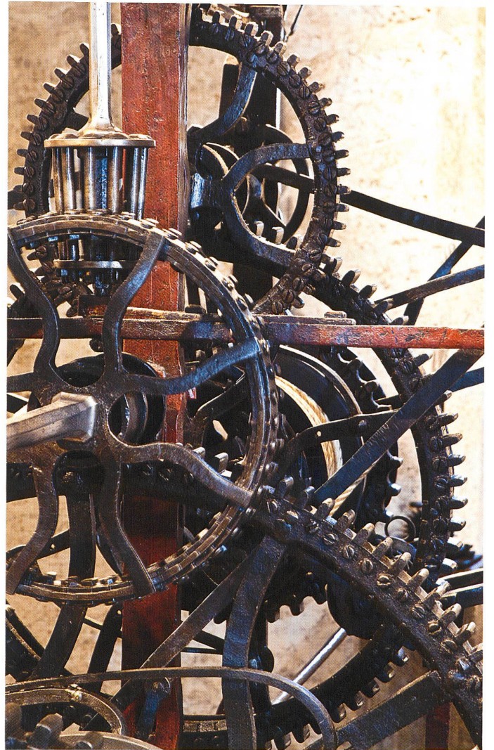
Zahnräder mit einzeln eingesetzten Zähnen
