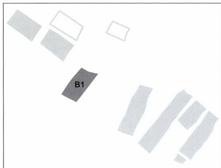
Fig. 11. Evolution chronologique et spatiale des unités architecturales pour la période B (phases H1, H2 et H3 à titre d'hypothèses).
