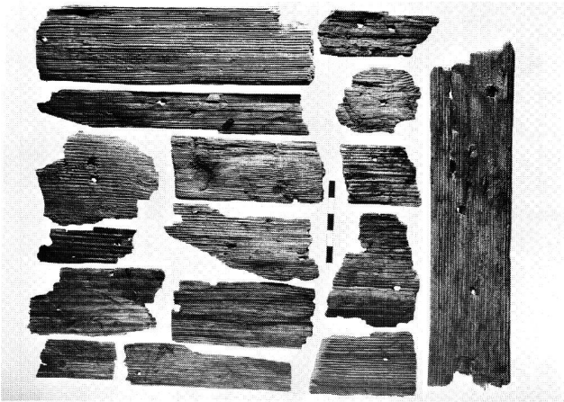
Abb. 49. Holderbank, Wässermatten, SO. Schindelfragmente mit Nagellochern. (Foto Eidgenössische Anstalt für das forstliche Versuchswesen, Birmensdorf.)
