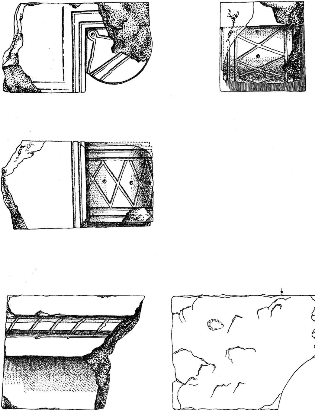
Abb. 51. Windisch AG, Oberburg 1956. Konsole und Gesims. – Maßstab 1:4.
