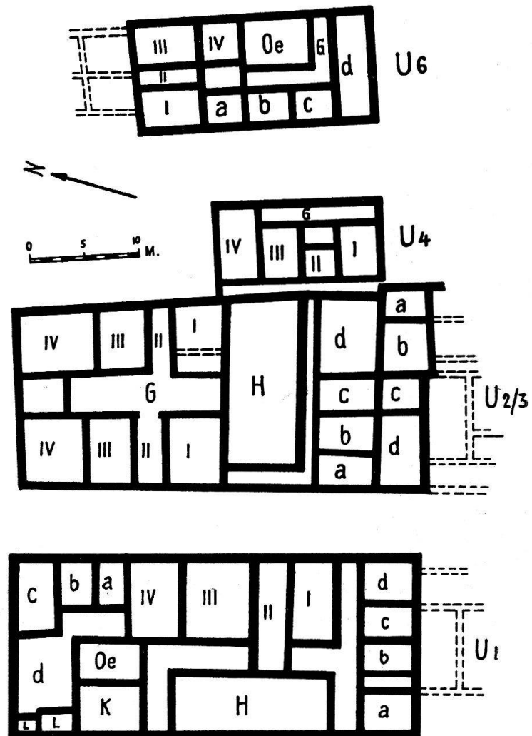
Abb. 8. Vindonissa. U.-O.-Häuser Schematischer Rekonstruktionsversuch (U 2/3 = Simonett U 2; U 4 = Sim. U 3; U 6 = Sim. U 5)
