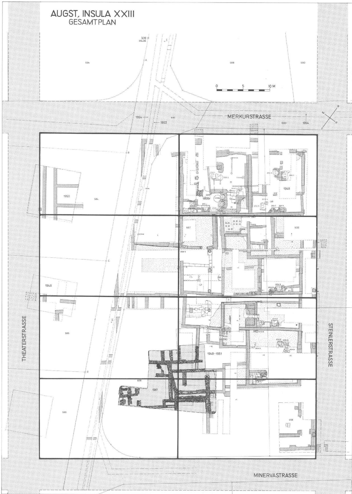
Abb. 2 Augst BL. Gesamtplan der Insula 23 mit vermutlicher Parzelleneinteilung (dicke Linien). Grabung 1987.56 durch steingerecht wiedergegebene Mauerzüge hervorgehoben. M. 1:400.
