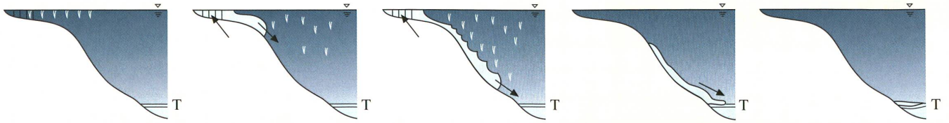
Von links nach rechts: Kaltes Wasser sammelt sich in Form von Zapfen an der Oberfläche. Am flachen Ufer kumuliert ebenfalls kaltes Wasser und rutscht wie eine Lawine nach unten ab. Gleichzeitig steigt warmes Wasser nach oben, wodurch Konvektionsschleifen entstehen. An der Thermokline (T-Niveau) erreicht die Kaltwasserlawine gleich temperiertes Wasser und löst sich auf.
