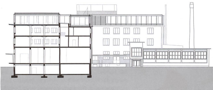
Längsschnitt
