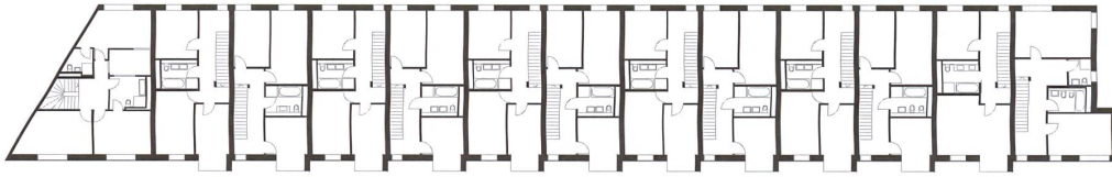
1. Obergeschoss Reihenhauszeile. | Maisons mitoyennes: 1 er étage.
