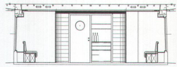
1-2 Schnitt durch die Buffet- und Treppeneinbauten, welche die beiden Decks des Motorschiffs «Zug» miteinander verbinden.
