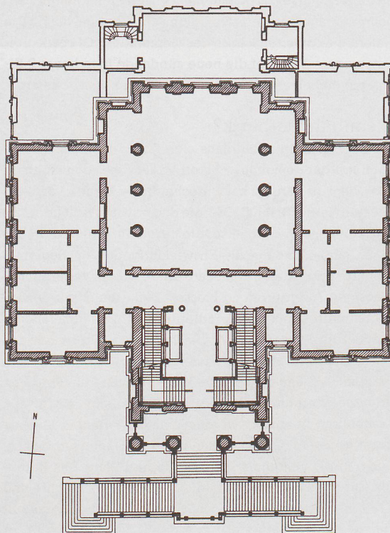
Grundriss des ersten Obergeschosses. Semper ursprünglicher Bau (schraffiert), Lebrecht Völkis Verlängerung (unschraffiert). Aus Peter Wegmann, Stadthaus Winterthur, Basel 1980
