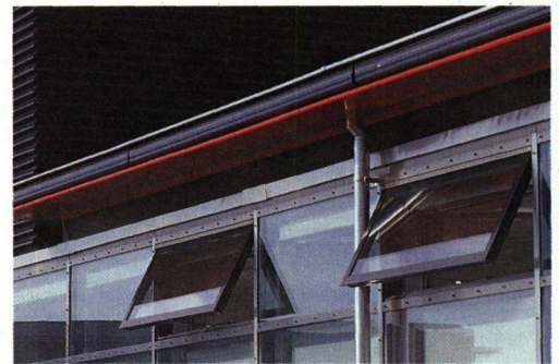
Punkt 2: Die Angestellten öffnen die Kippfenster, um nachts die Betondecke zu kühlen
