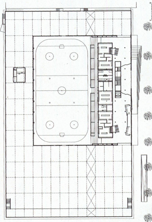
Grundriss Erdgeschoss
