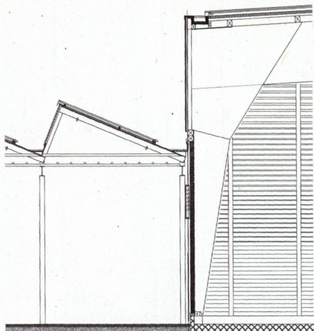
Detailschnitt Eishalle-Viehmarkthalle
