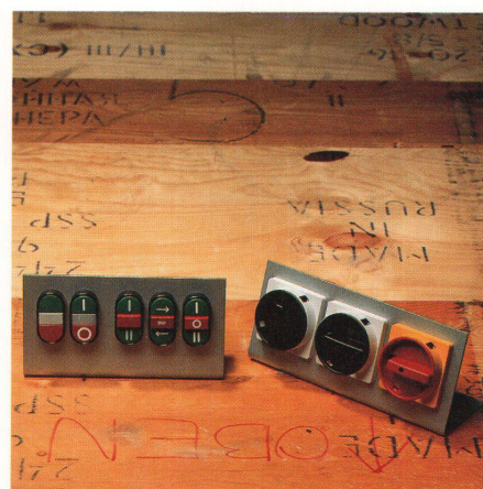
Produkt: Multifunktionstaste DM 3 und Haupt-Notausschalter L2 (rechts) Design: Fernand Hofer, Sprecher + Schuh Werkdesign, Aarau Hersteller: Sprecher + Schuh, Aarau
