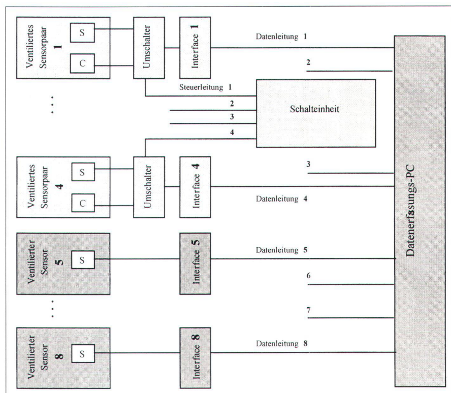
Abb. 3: Aufbau des Messsystems (S = Standardsensor; C = Chipausführung).
