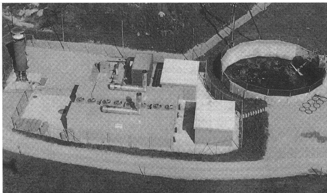
Abb. 4: Deponiegas-Verstromungsanlage Ufhusen.
