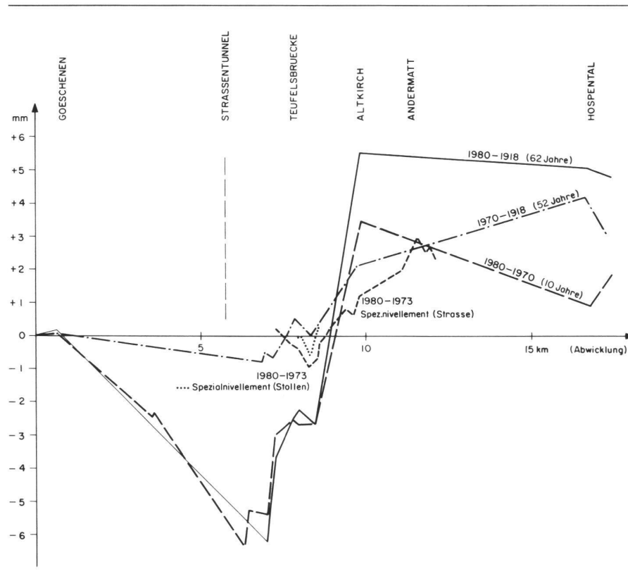
Abb. 5 Nivelllements der L+T von 1918 bis 1980 in den Schöllenen.
