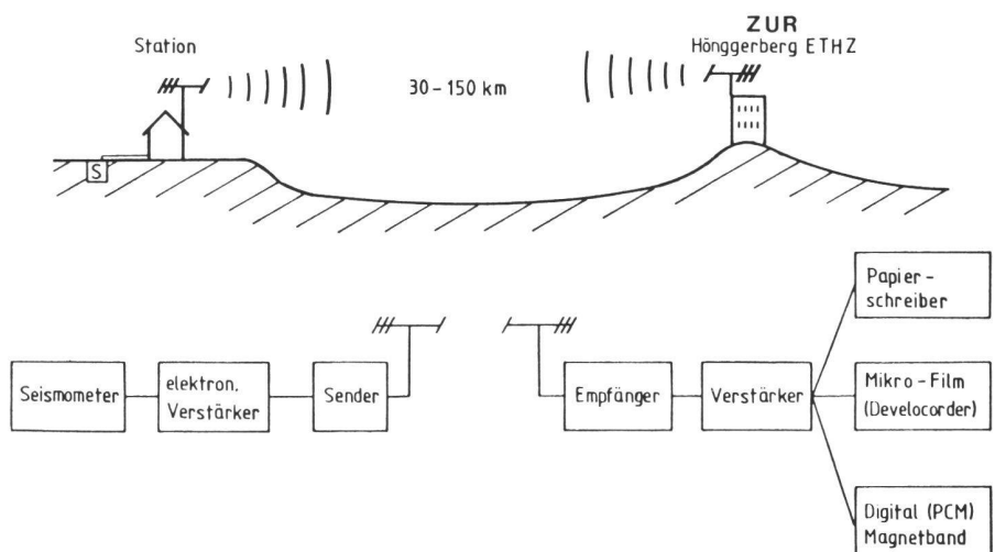
Abb. 11 Blockscheema der Fernübertragung seismischer Signale vom Seismometer S bis zur Registrierzentrale in der ETH-Hönningerberg.
