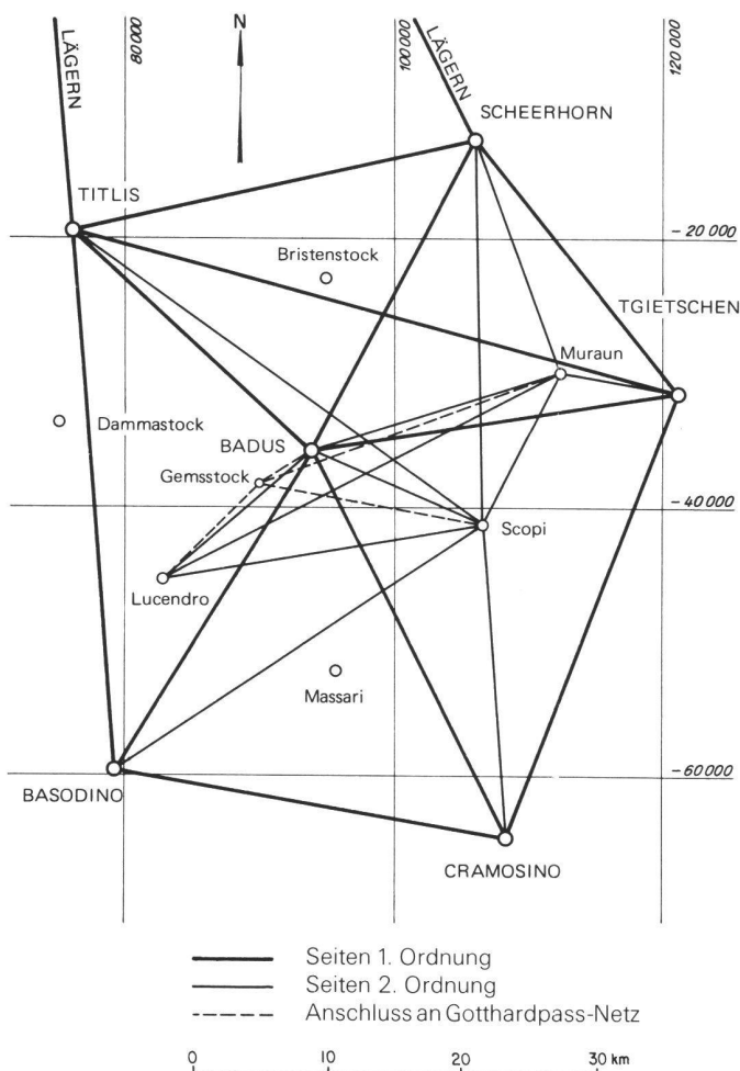
Abb. 8 Testnetz Gotthard
