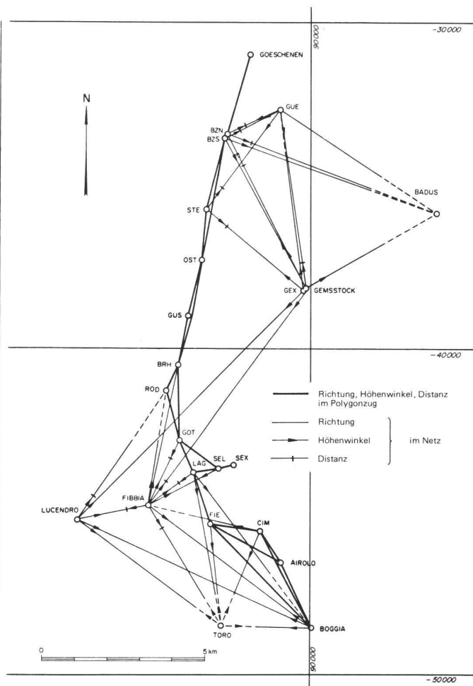
Abb. 9 Gotthardpass-Netz
