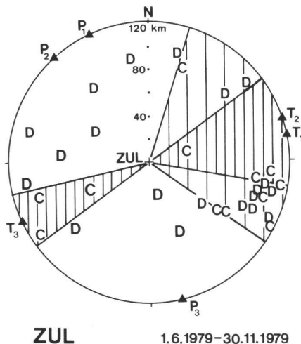
Abb. 13 Stations-Diagramm für die Erdbebenstation Zürich-Lägeren ZUL des Schweiz. Erdbebendienstes. Das Diagramm veranschaulicht die Verteilung von Kompression (C) und Dilatation (D) für Nahbeben bis 120 km Epizentraldistanz, registriert an der Station ZUL in der Zeit vom 1. Juni 1979 bis 30. November 1979. Die Art des an der Station beobachteten Erst-Einsatzes der P-Wellen (Kompression oder Dilatation) wird im Diagramm dort eingetragen, wo von der Station aus gesehen nach Azimut und Distanz das Epizentrum des betreffenden Bebens liegen würde (Pavoni, 1982). Es lassen sich Sektoren mit Kompression C (eng schraffiert) und Dilatation D sowie Übergangsbereiche mit Kompression und Dilatation (weit schraffiert) abgrenzen. P und T markieren die Azimute für die Orientierung der Achsen der maximalen und minimalen horizontalen Hauptspannungen in der oberen Kruste in der Umgebung der Station ZUL.
