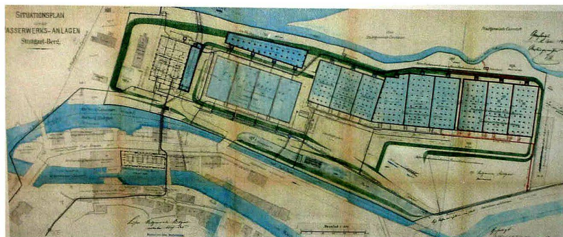
Lageplan des Neckarwasserwerks Berg. Die Anlage war durch einen Schuttdamm (in Grün) gegen den noch nicht verbauten Neckar geschützt. Die zahlreichen Kanäle beziehungsweise Seitenarme des Neckars trieben eine Vielzahl von Wasserrädern im «Mühlenstandort» Berg.
