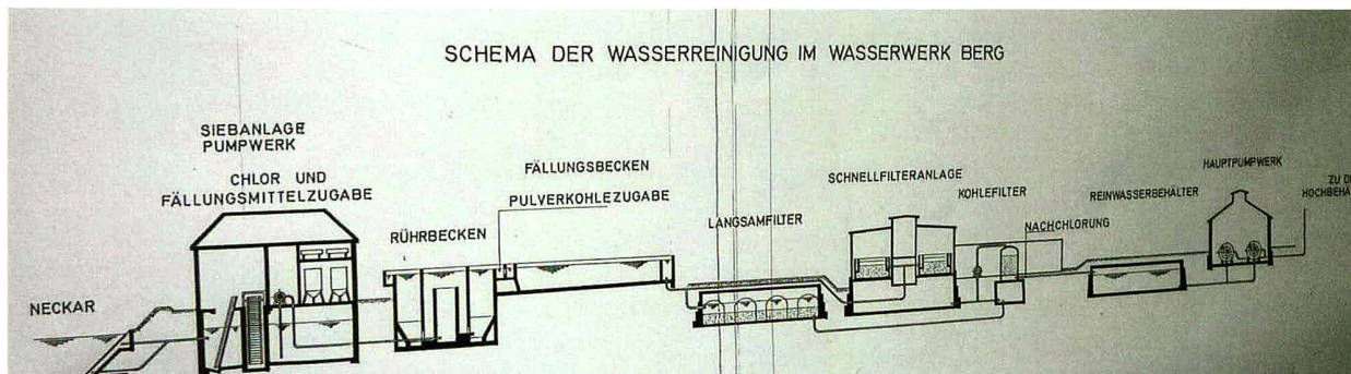
Funktionsschema, kommentiert (Objekterklärung beim Tag der offenen Tür, Februar 2011).
