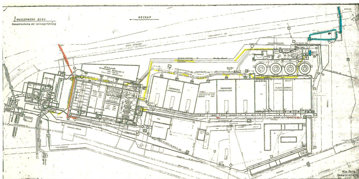
Lageplan um 1930 (Objekterklärung beim Tag der offenen Tür, Februar 2011).
