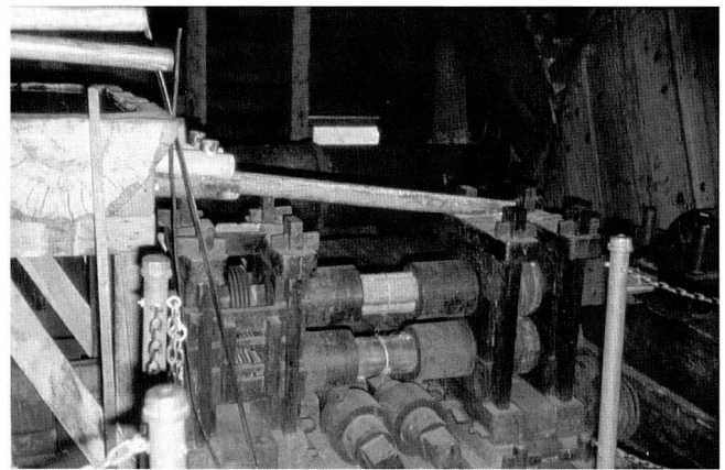
Walz- und Schneidewerk der Saugus Ironworks, etwa 1790 (erstmals um 1650).
