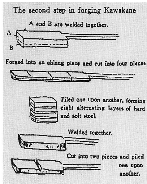
Schema der japanischen Damaszener-Techniken (nach Chikashige, o.c.)
