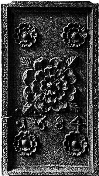
Ofenstirnplatte mit Rosettenornamentik. bez. 1684. Harz oder Sachsen. Abm. 60,0 x 34,5 cm
