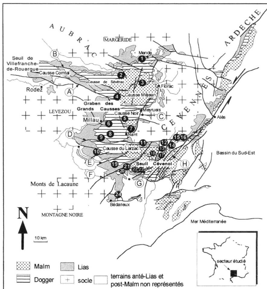
Fig. 1. Carte géographique et géologique de la région étudiée et localisation des affleurements cités (1: Changevèze; 2: La Canourgue; 3: Chambonnet; 4: Les Vignes; 5: Montméjean; 6: Millau; 7: Saint-Sulpice; 8: La Cavalerie; 9: Saint-Rome-de-Cernon; 10: Saint-Beaulize; 11: Aurières; 12: Horst de Saint-Bresson; 13: Les Malines; 14: Les Avinières; 15: Sumène; 16: Col du Lac; 17: Gornières; 18: Le Viala; 19: Le Clapier; 20: Labeil; 21: Pas de l'Escalette; 22: Cirque du Bout du Monde; 23: Saint-Pierre-de-la-Fage; 24: Bédarieux; A: faille des Palanges; B: faille de Coussergues, faille du Pas de Soucy; C: faisceau de Meyrueis; D: faille de l'Hospitalet; E: faille de La Pezade; F: faille de Saint-Martin; G: faisceau de la Vacquérie; H: faisceau cévenol).
